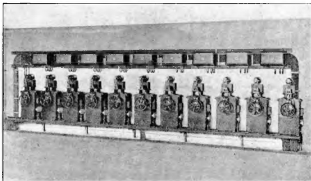
Automatische schakelinrichting of wel tijdrelais.
