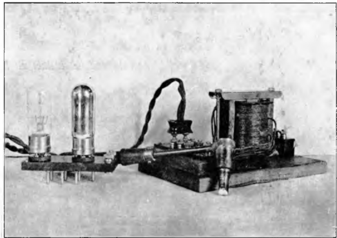
Model-transformator vervaardigd volgens bovenstaande gegevens.
