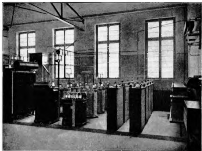
Afvlak-inrichting der gelijkrichter-installatie.
